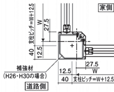
●90°コーナー専用柱
