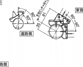
●出隅(鋭角)の場合
